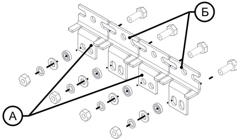
Рис. 1 Козырек защитный шкафов UC2.
