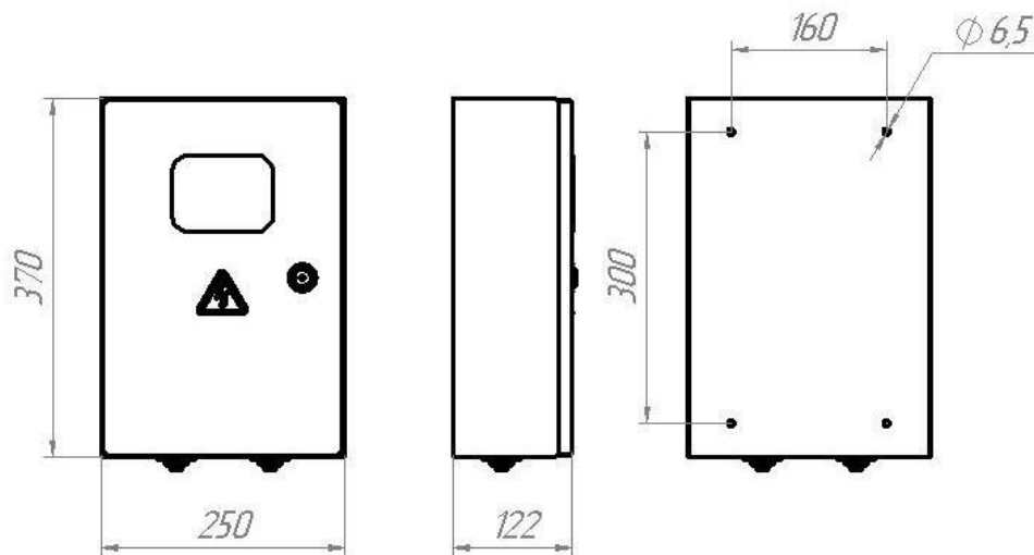
Рис. 1 Габаритные и установочные размеры.
